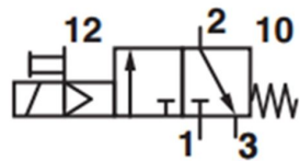
Válvula 3/2 solenoide resorte
