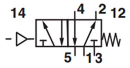
Válvula 5/2 aire resorte
