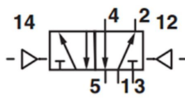
Válvula 5/2 aire aire
