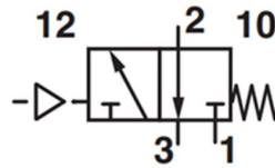
Válvula 3/2 aire resorte NC
